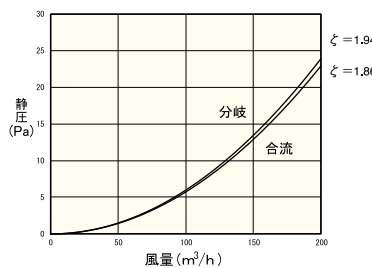
■ 圧力損失曲線 (ADF-060T75)
