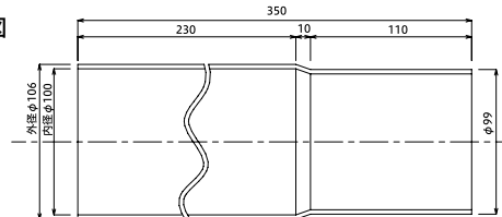
φ100 塩ビ絞り管 L=350 AS-100S (コード/GYB01798) 価格：2,750円/個 (税抜価格 2,500円)
