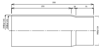
φ125 塩ビ絞り管 L=350 AS-125S (コード/GYB01799) 価格：5,390円/個 (税抜価格 4,900円)
