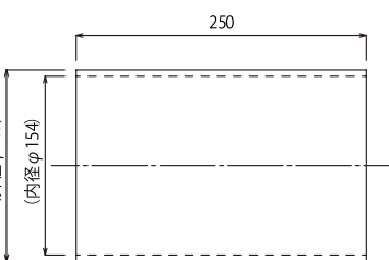
φ150 塩ビ管 L250 AS-150-250 (コード/GYB01793) 価格：2,750円/個 (税抜価格 2,500円)
