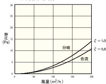
■ 圧力損失曲線 (ADF-060T75)
