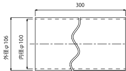
φ100 塩ビ管 L300 AS-100-300 (コード/GYB01792) 価格：1,430円/個 (税抜価格 1,300円)
