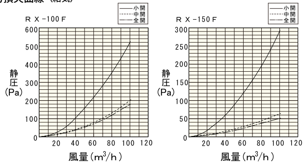
■圧力損失曲線 (給気)
