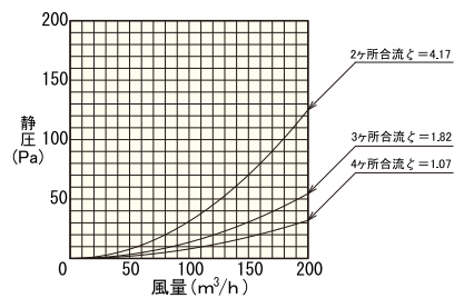
■ 圧力損失曲線 (合流)
