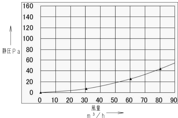
圧力損失曲線（吸込） \zeta = 1.08
