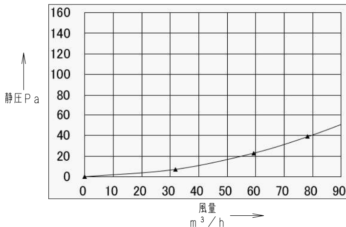
圧力損失曲線（吹出） \zeta = 1.01
