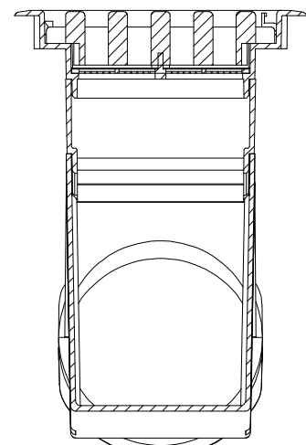
断面図A-A
